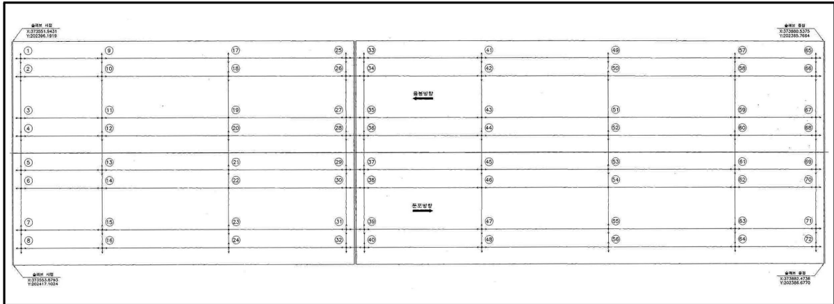
<그림 6.14> 받침배치도
