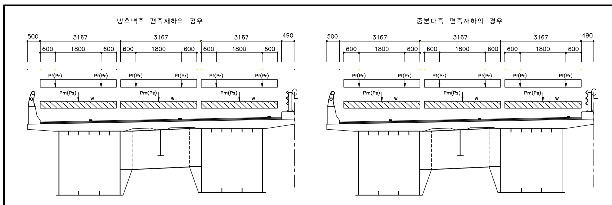
〈그림 6.7〉 설계활하중 재하의 경우
