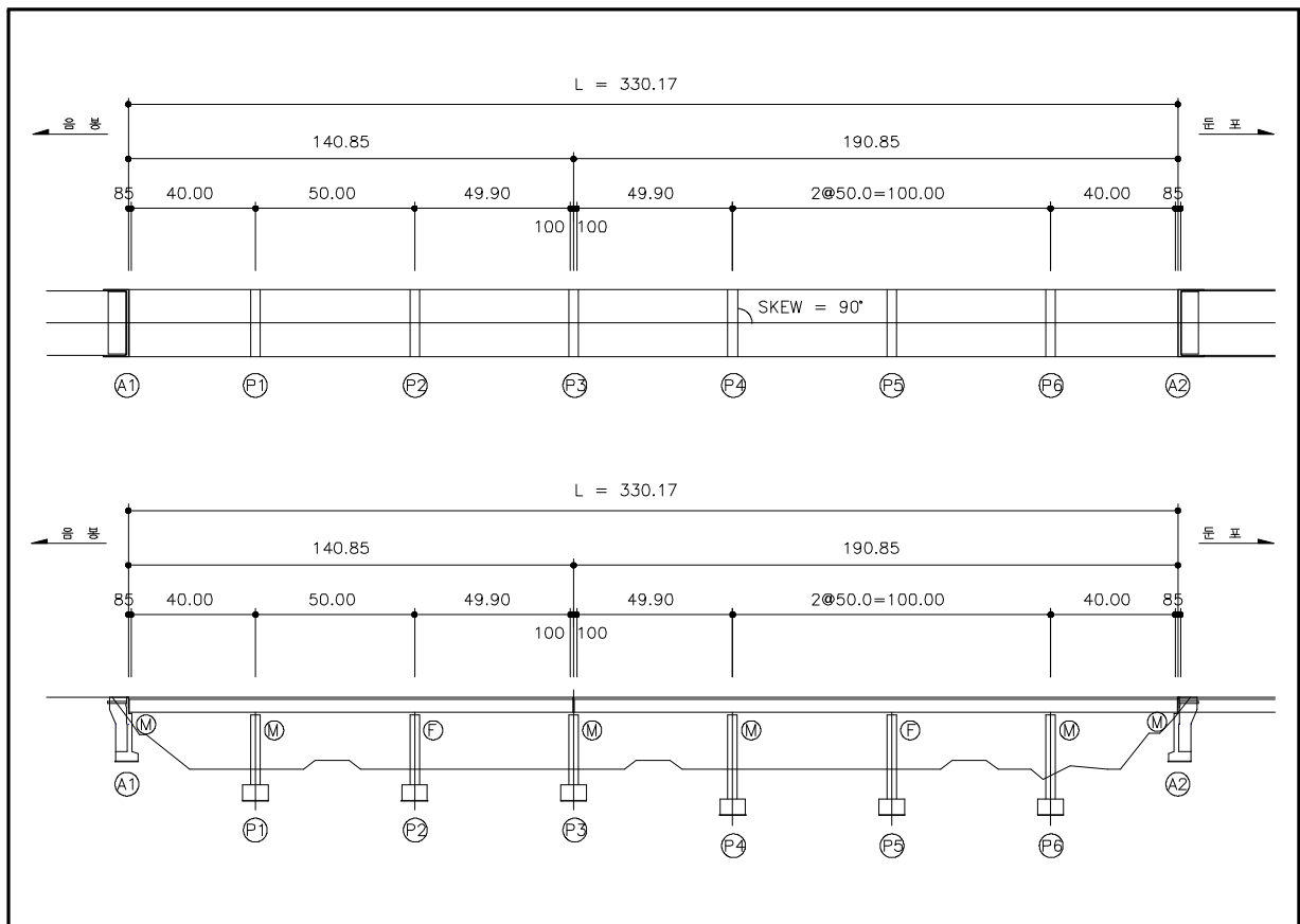
<그림 6.1> 원남교(하) 종평면도
